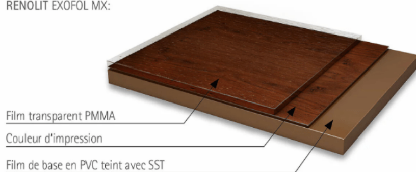
Structure schématique de la feuille extérieure RENOLIT EXOFOL MX:
