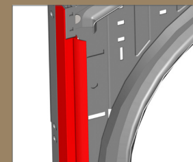
JOINT À LÈVRES VERTICAL
