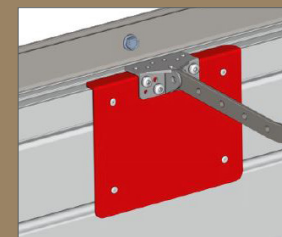
PLAQUE RENFORT ACCROCHE MOTEUR
