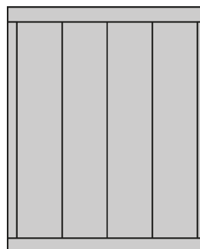
RAINURES VERTICALES PAS DE 250MM
