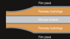
Double isolation phonique et thermique
