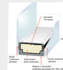
Coupe de l'intercalaire Warm Edge
