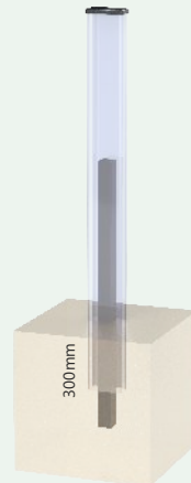
POTEAU 76x41 à sceller direct avec tube 30x30 acier Longueur 1.500mm Hauteur maxi conseillée 1.800mm
